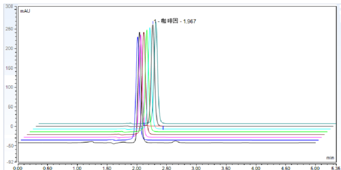
图 D.1 40 µg/ml 咖啡因标准溶液保留时间及精密度核查色谱图 (n=8)
