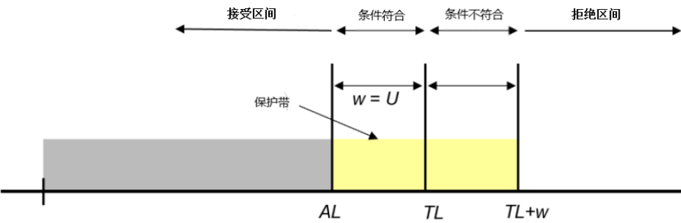
图 B.2 基于保护带 w=U 的非二元接受图示
