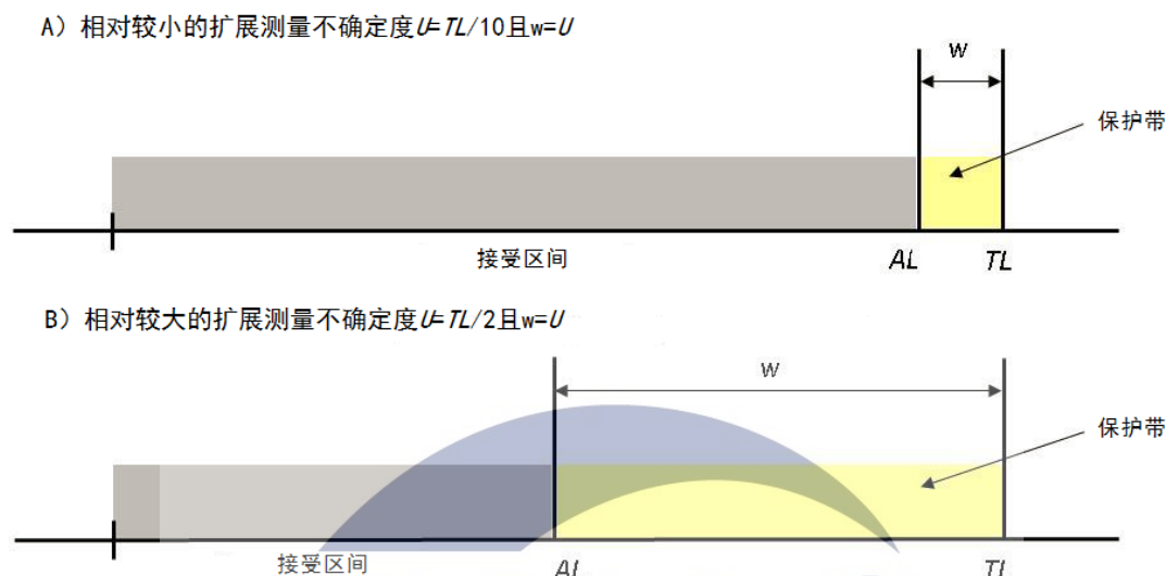
图 6 不同长度的保护带对应的接受区间
