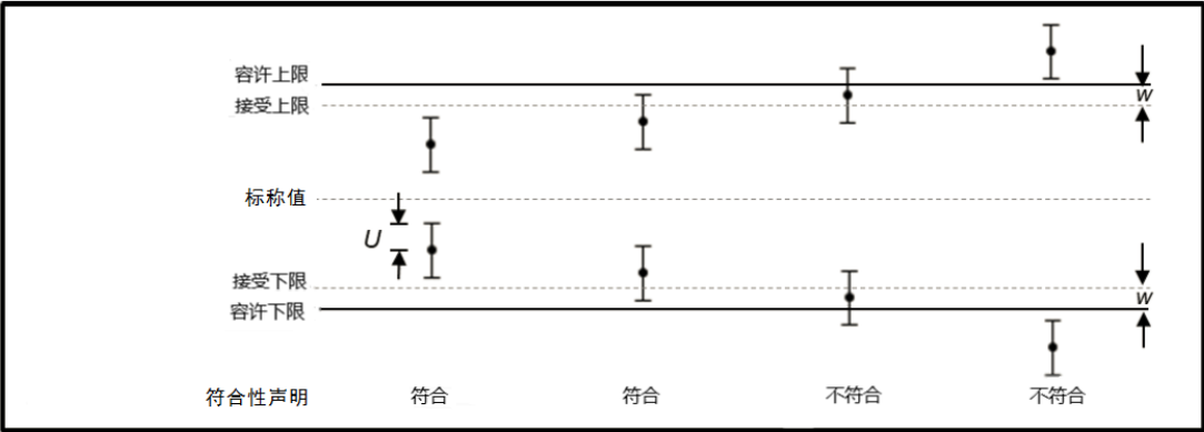
图 4 有保护带的二元判定规则图示（ w=U ）
